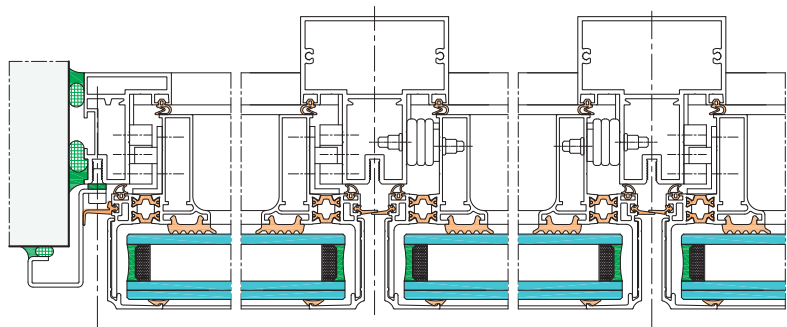
Coupe horizontale
